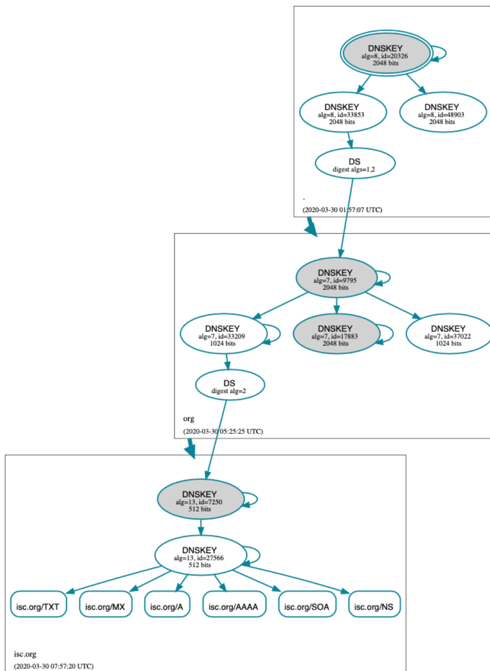
Fig. 4: DNSViz
